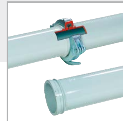
Sistema de acoplamiento estándar SK
